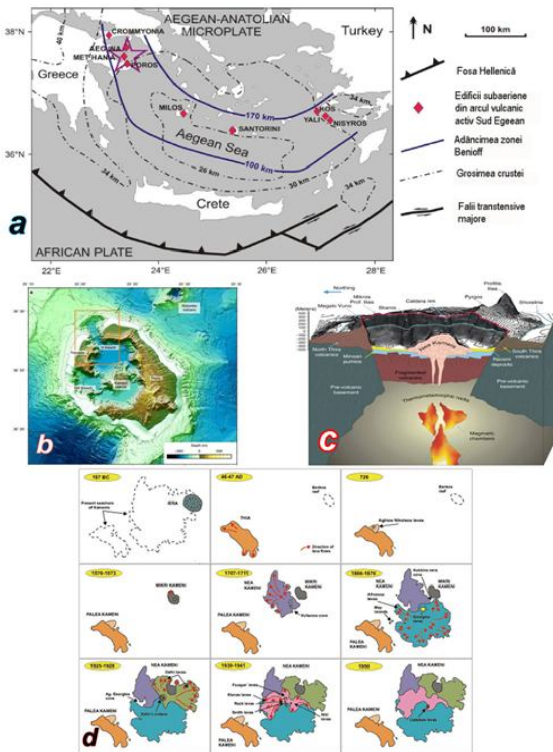
Fig. 2. - a. Edificiile vulcanice din arcul Aegean (Hellenic) și configurația crustei (după Bayley et al., 2009); - b. Modelul 3D al edificiului vulcanic Santorini (după Gorocovich, 2013); - c. Secțiune prin edificiul vulcanic Santorini (după Gorocovich, 2013); - d. Evoluția vulcanismului postminoic din Santorini - Palea și Nea Kameni (după ISMSV, ),
