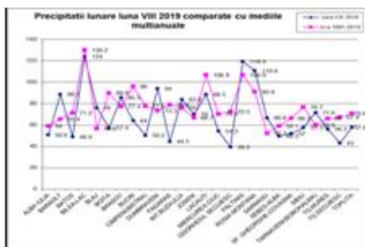
Fig. 3 a) Graficul temperaturilor medii, luna august 2019 comparativ cu mediile multianuale de referință (1981-2010); b) Harta abaterii temperaturii medii, luna august, față de mediile multianuale (1981-2010, după ANM București); c) Harta cu repartitia izotermelor la nivelul Europei (după www.wetterzentrale.de ); d) Graficul precipitațiilor, luna august 2019 comparativ cu mediile multianuale de referință (1981-2010); e) Harta abaterii cantității lunare de precipitații, luna august 2019, față de mediile multianuale (1981-2010 după ANM București).
