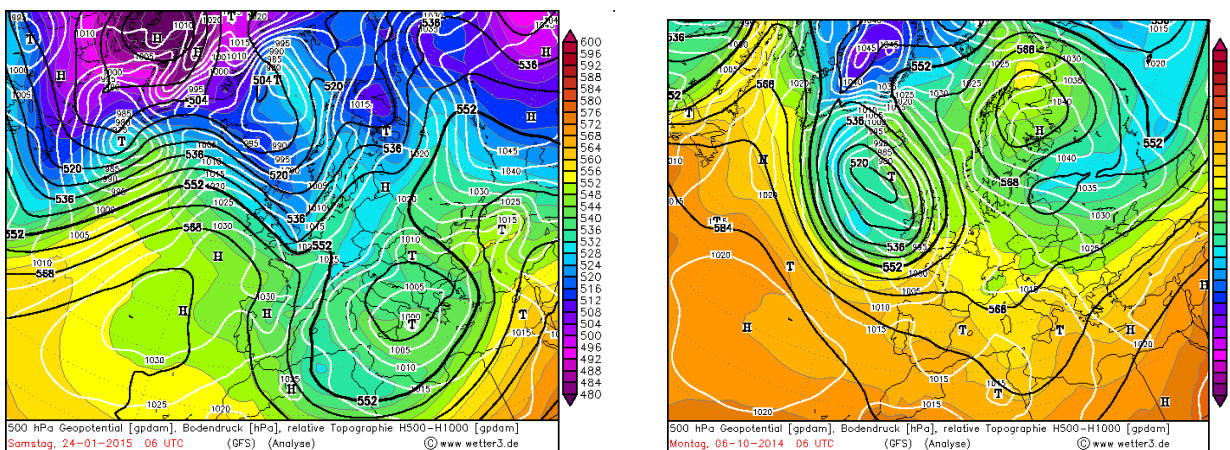
Fig. 3 a) Presiunea la sol(hPa) -linii albe, 24.01.2015 06 UTC; b) Presiunea la sol(hPa) -linii albe, 06.10.2014 06 UTC
