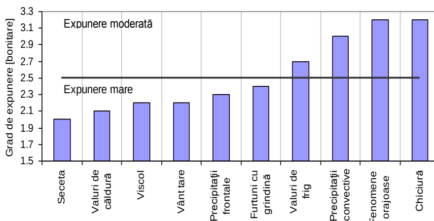
Fig. 1, Expunerea regiunii Câmpiei Române la fenomene meteorologice periculoase (în grade medii de bonitare).
