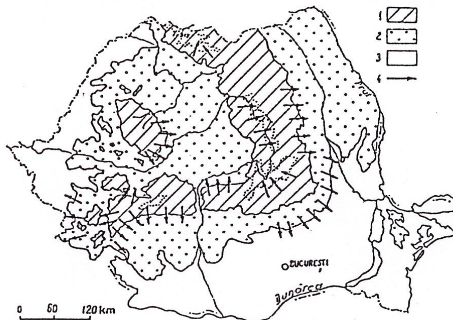
Fig. 1, Fohnul carpatic (după Bogdan, 1993)
