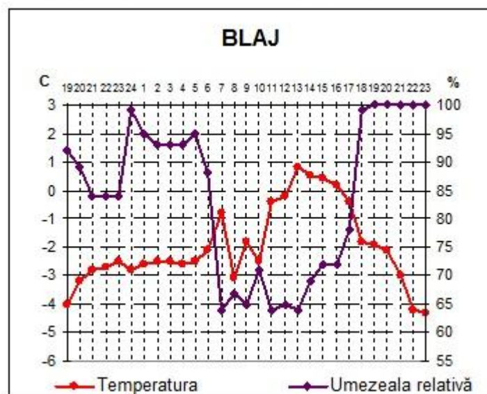
Fig. 3b, Evoluția temperaturii și umezelii relative a aerului, în intervalul 17-18. 01. 2000.
