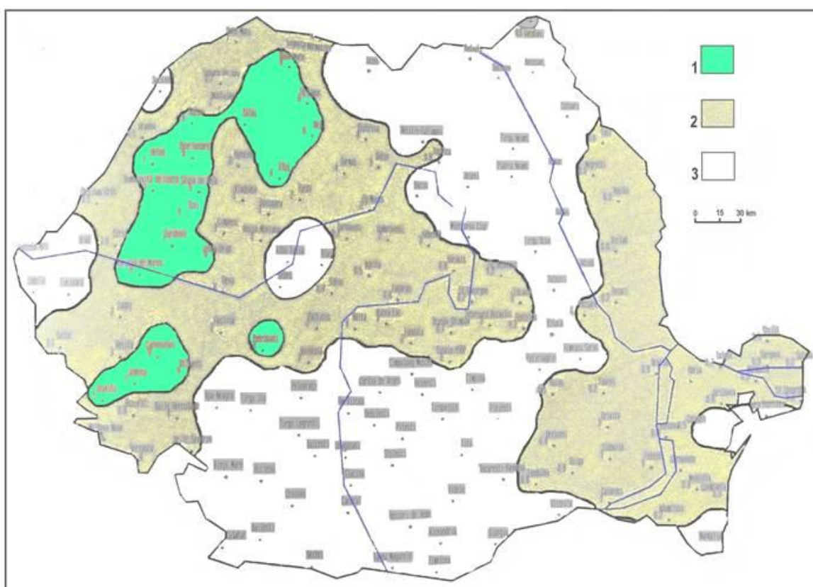
Fig. 3a, Harta repartiției precipitațiilor în 18.01.2000, la ora 2: 1, >5 mm; 2, 0.1 - 5 mm; 3, 0 mm (după Arhiva sinoptică ANM).
