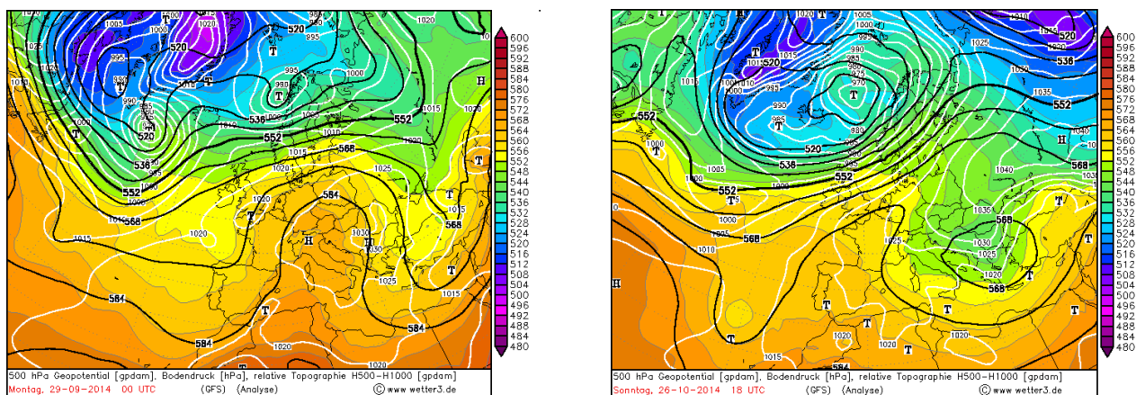
Fig. 1 a) Presiunea la sol(hPa) -linii albe, 29.09.2014 00 UTC; b) Presiunea la sol(hPa) -linii albe, 26.10.2014 18 UTC
