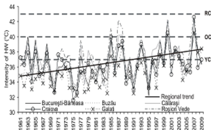
Fig. 5, Variabilitatea intensității absolute a valurilor de căldură extreme (Dragotă, Havriș, 2015)
