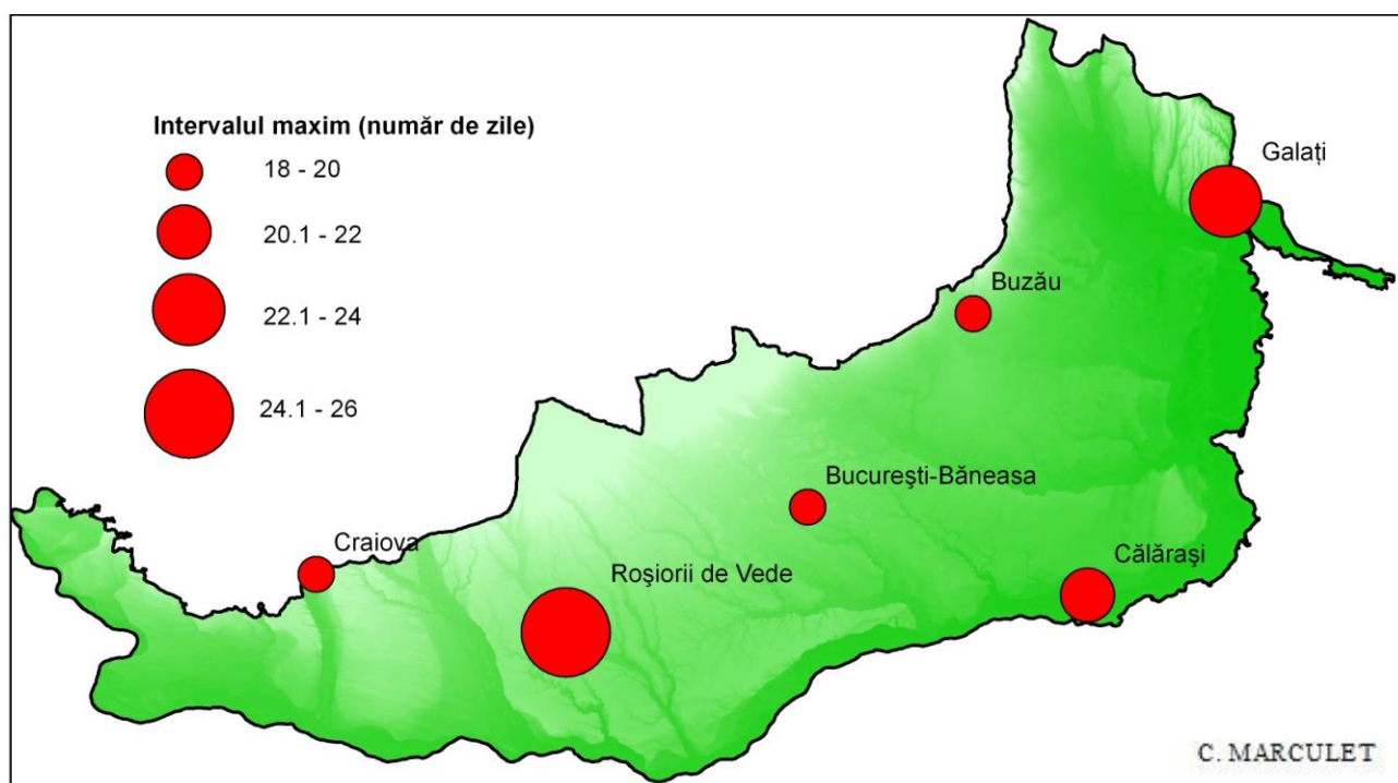
Fig. 7, Harta distribuției duratelor maxime ale intervalurilor simultane cu zile tropicale și fără precipitații din lunile de vară (1961-2009).
