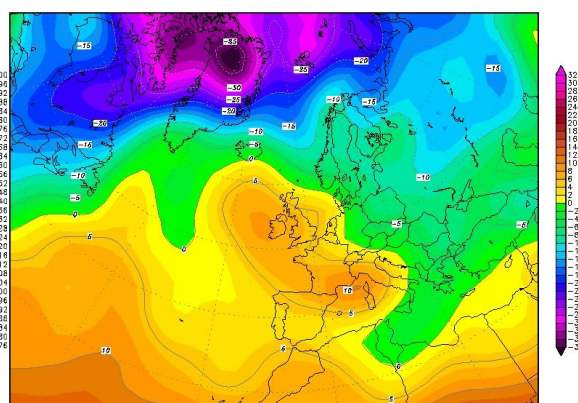
Fig. 2b, Temperatura (°C) la 850 hPa (8500 m), 18.01.2000, ora 00 GMT (din arhiva Centrului Meteorologic Karlsruhe)
