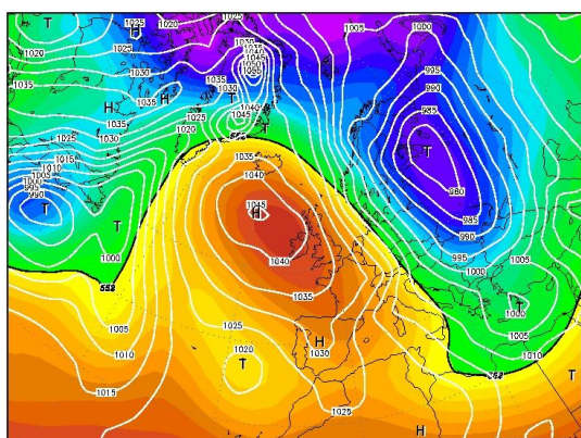
Fig. 2a, Câmpul presiunii atmosferice la sol și câmpul de geopotential la 500 hPa (5500 m), 18.01.2000, ora 00 GMT (din arhiva Centrului Meteorologic Karlsruhe)
