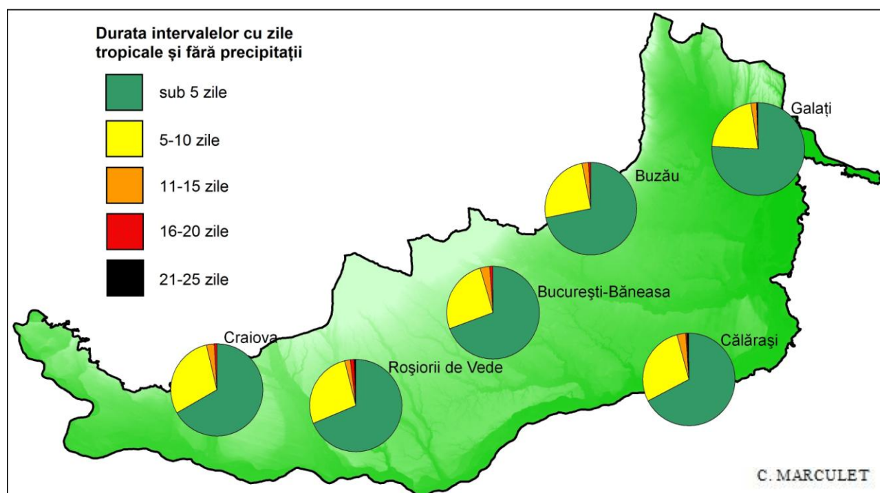
Fig. 6, Harta distribuției pe praguri de valori a zilelor consecutive tropicale în cuplaj cu cele fără precipitații din lunile de vară (1961-2009).
