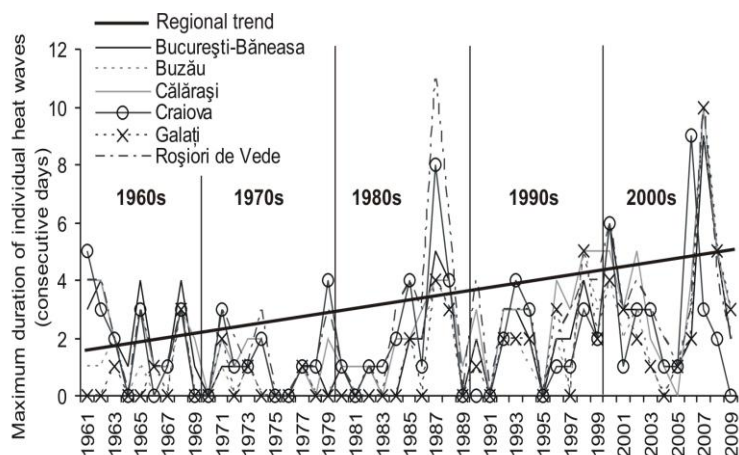
Fig. 4, Variabilitatea duratei maxime a valurilor de căldură individuale în Câmpia Română (Dragotă, Havriș, 2015).
