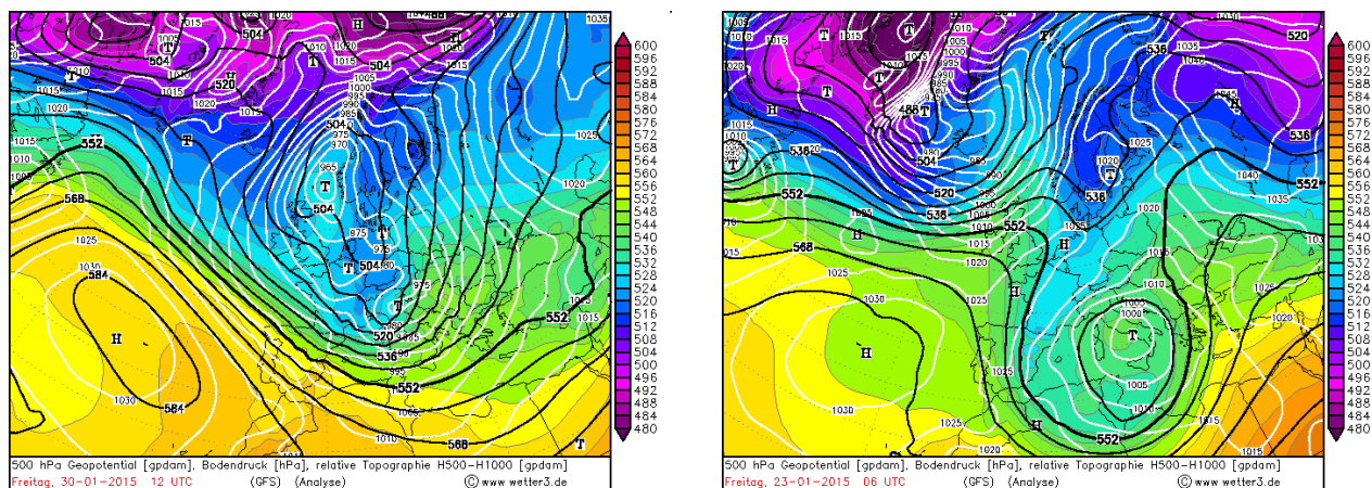
Fig. 2 a) Presiunea la sol(hPa) -linii albe, 30.01.2015 12 UTC; b) Presiunea la sol(hPa) -linii albe, 23.01.2015 06 UTC
