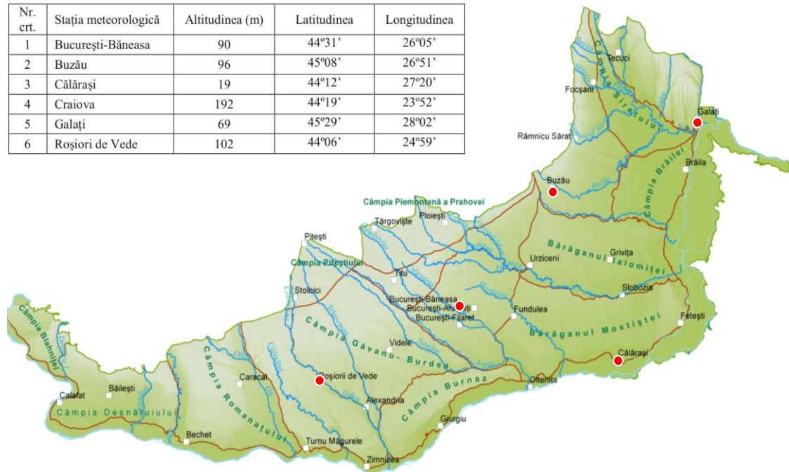
Fig. 2, Coordonatele geografice ale stațiilor meteorologice ECA&D din Câmpia Română.
