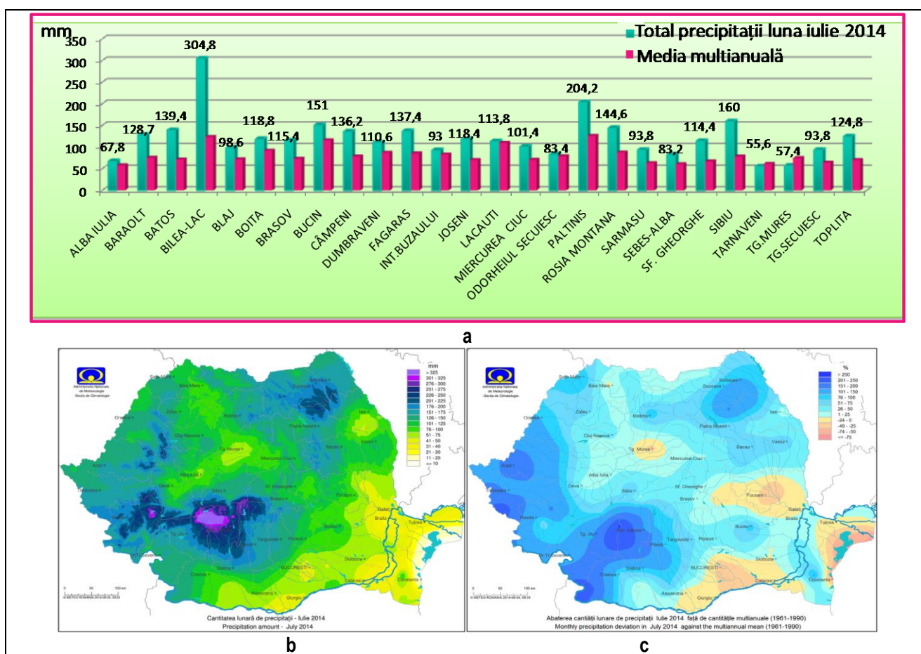
Fig. 3. a) Graficul precipitațiilor din luna iulie 2014, comparativ cu mediile multianuale (mm), b) Harta cu repartitia la nivelul României a precipitațiilor medii lunare (iulie 2014) (*după ANM), c) Harta cu abaterea precipitațiilor medii lunare (iulie 2014), față de mediile multianuale) (*după ANM).
