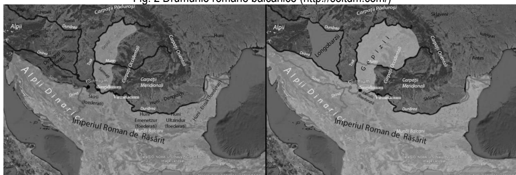
Fig. 3 Hărțile reprezintă două perioade: 458-469 și 536-567
