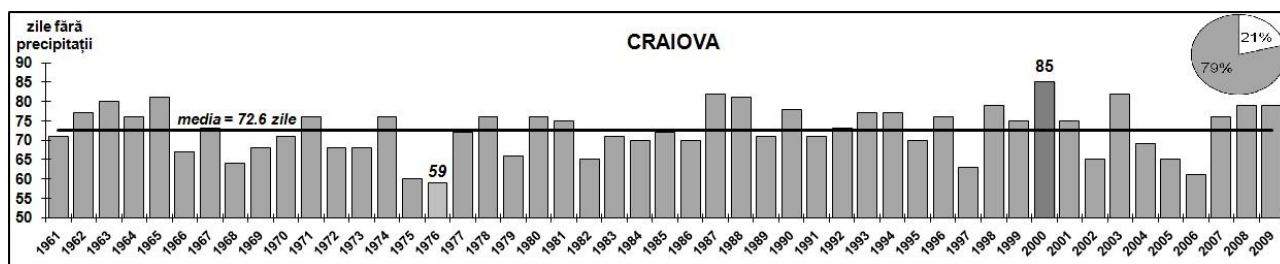
Fig. 2, Variația anuală a numărului de zile fără precipitații în anotimpul de vară și proporția acestora din totalul zilelor calendaristice (1961-2009), în Câmpia Olteniei.
