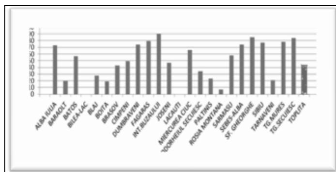
Fig. 1. Graficul cu numărul de cazuri de brumă din intervalul 2004-2013: a) luna august, b) luna iunie, c) luna septembrie, d) luna octombrie, e) luna mai, f) luna aprilie, g) luna martie.
