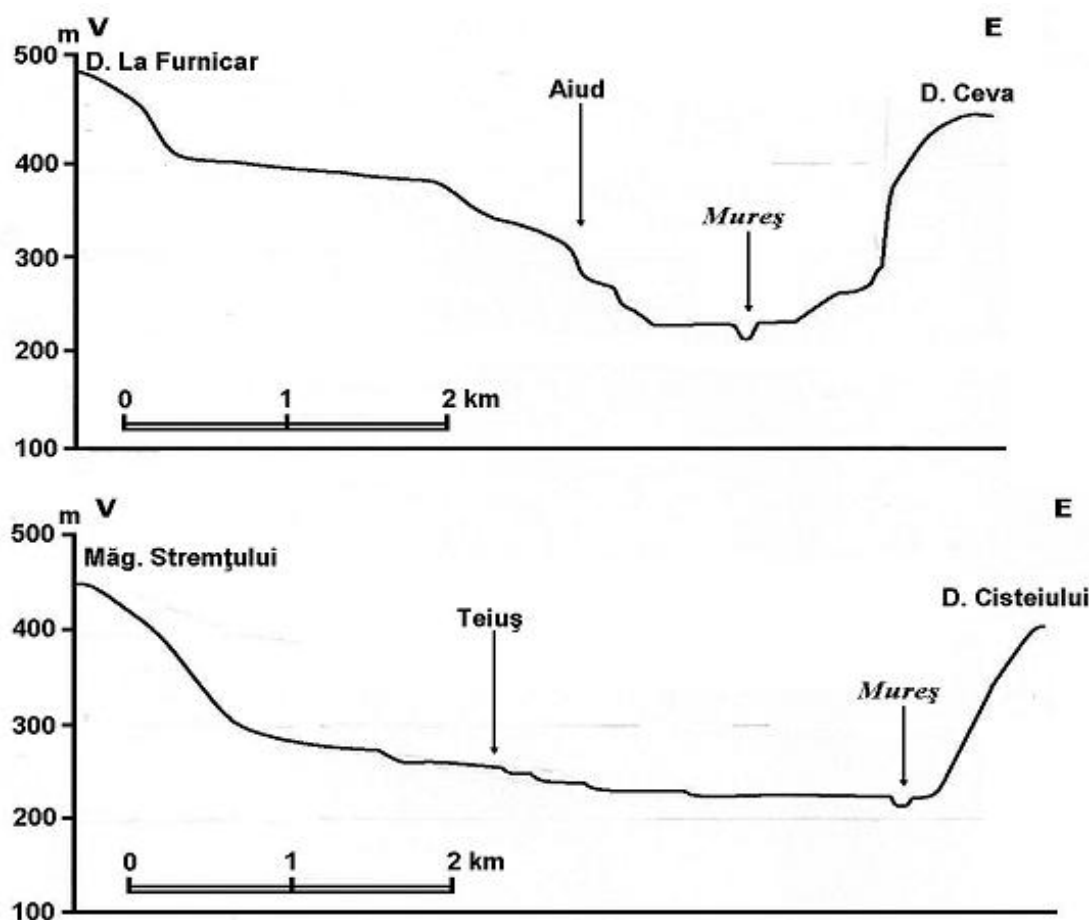
Fig. 1. Profile transversale la Aiud și Teiuș
