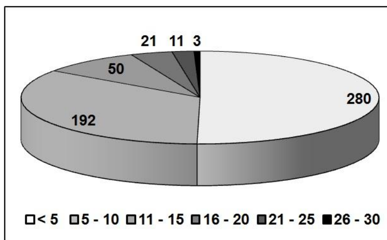
Fig. 3, Frecvența absolută pe clase de valori a duratei intervalelor de zile consecutive fără precipitații din lunile de vară, în Câmpia Olteniei (1961-2009).
