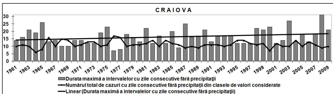
Fig.4, Variația intervalelor cu zile consecutive fără precipitații din anotimpul de vară (1961-2009).
