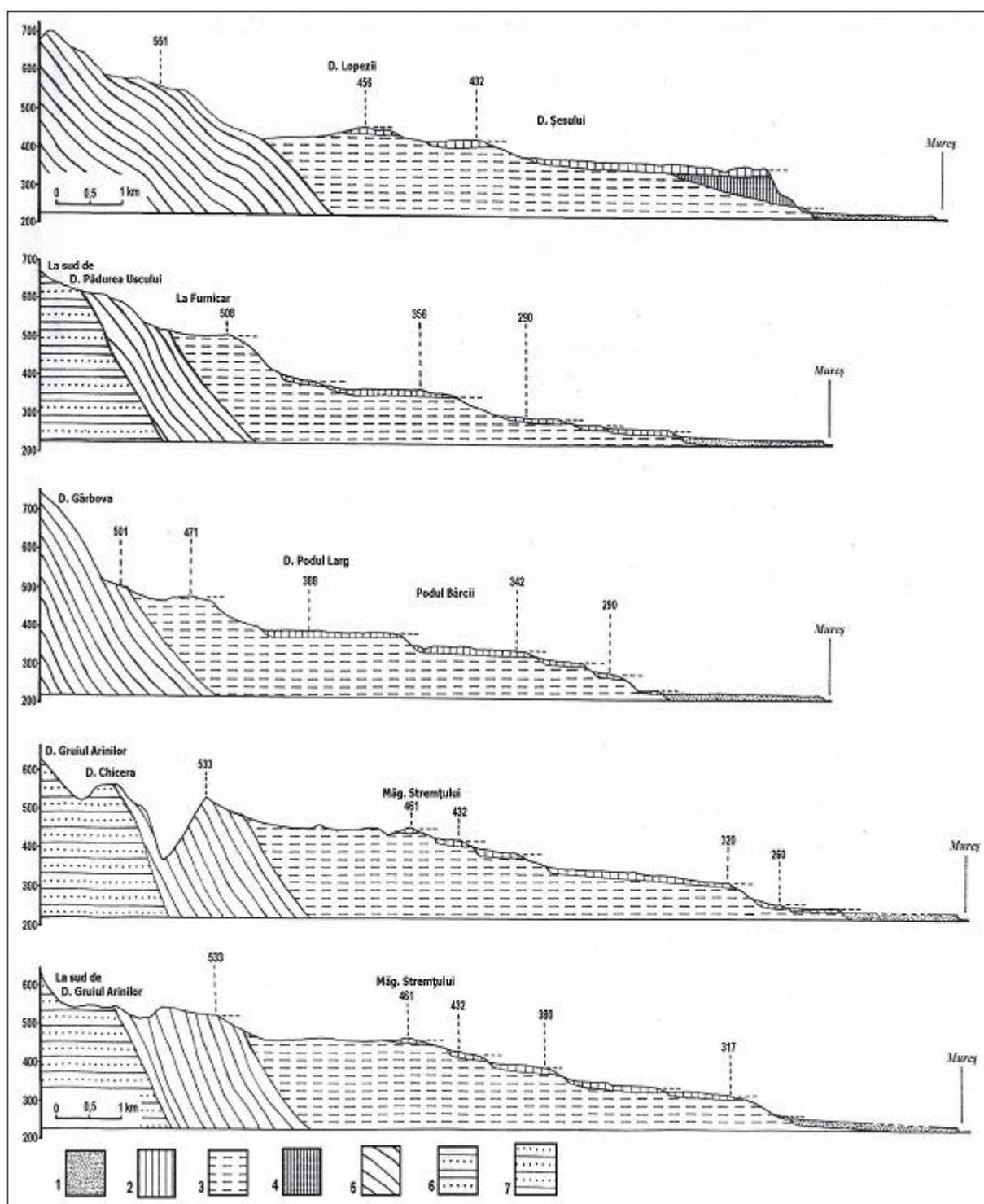
Fig. 2. Profile transversale geologice prin Culoarul Mureșului între Aiud și Alba Iulia: 1, luncă; 2, terase; 3, Pannonian; 4, Sarmatian; 5, Badenian; 6, Cretacic inferior; 7, Cretacic superior.
