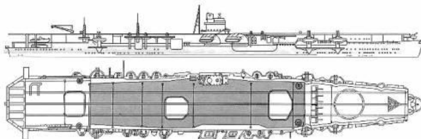
Profilul portavionului japonez „Hiryū”. (sursa: http:// forum.worldofwarships.eu 11)
