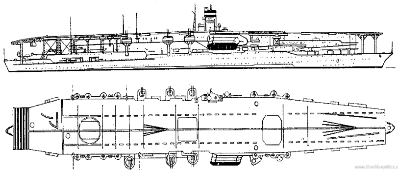
Profilul portavionului japonez „Akagi”, nava – amiral a Kido Butai .
