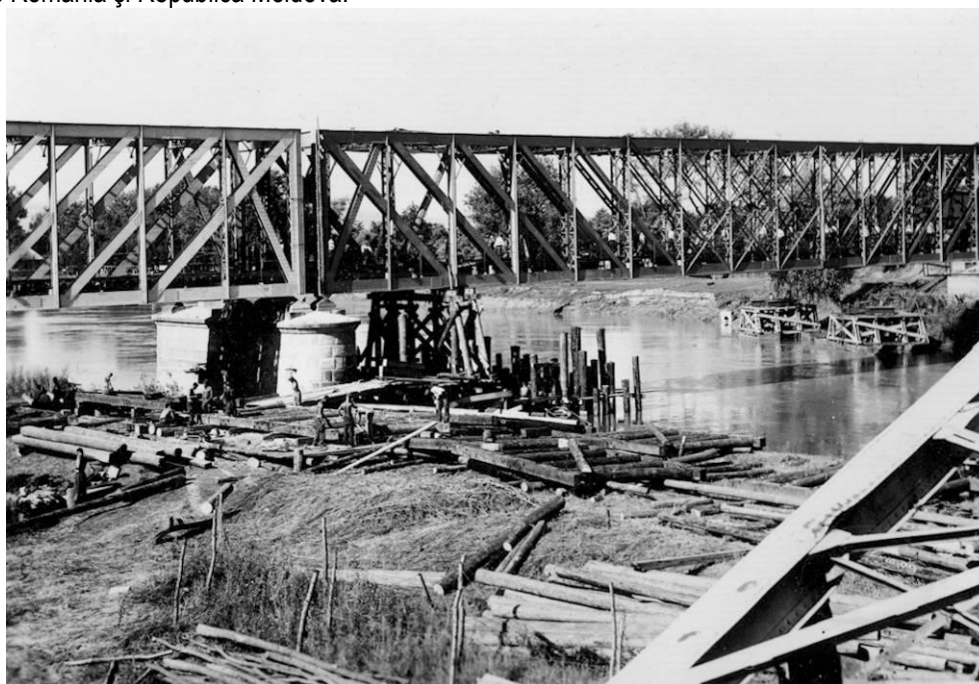
Fig. 2 Consolidarea podului feroviar de la ieșirea din stația Ungheni – 1941
