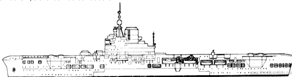
Profilul portavionului britanic „HMS Illustrious”.
