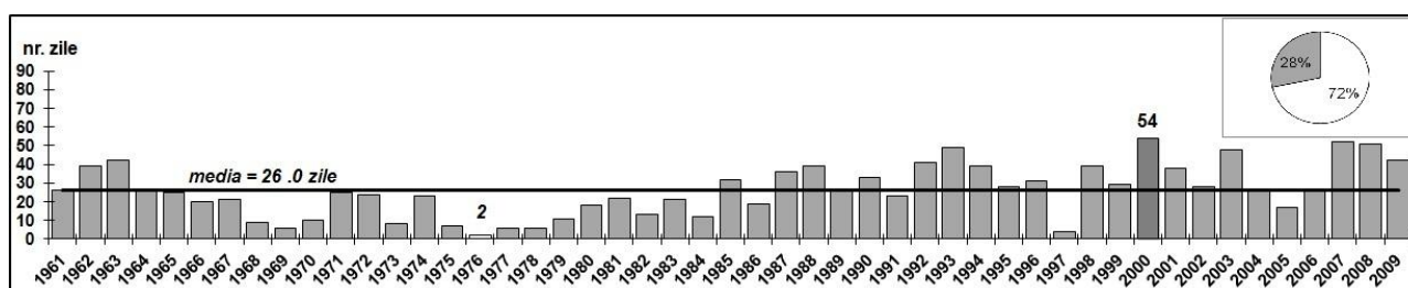
Fig. 8, Variația numărului total de zile simultane cu temperaturi tropicale și fără precipitații, din anotimpul de vară, raportate la numărul total al zilelor calendaristice (1961-2009), în Câmpia Olteniei.
