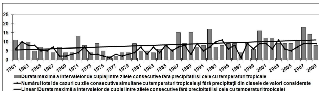
Fig. 10, Variația simultaneității zilelor consecutive cu temperaturi tropicale și cele fără precipitații din anotimpul de vară (1961-2009) în Câmpia Olteniei.
