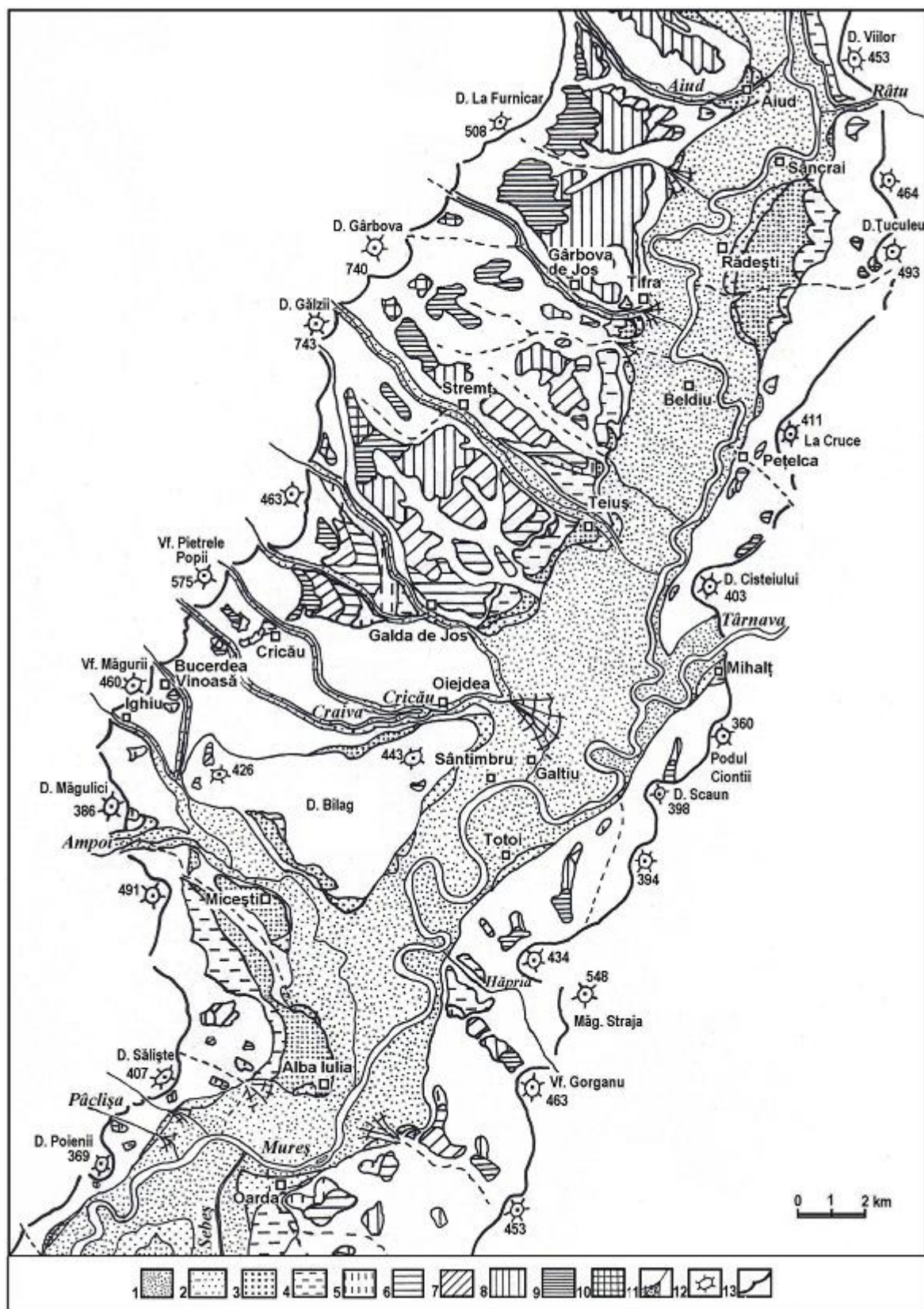
Fig. 3. Harta teraselor Mureșului din Culoarul Aiud – Sebeș: 1, lunca; 2, terasa 1-a (6-9 m altitudine relativă); 3, terasa a 2-a (12-15 m alt. rel.); 4, terasa a 3-a (18-25 m alt. rel.); 5, terasa a 4-a (30-40 m alt. rel.); 6, terasa a 5-a (50-60 m alt. rel.); 7, terasa a 6-a (72-80 m alt. rel.); 8, terasa a 7-a (90-110 m alt. rel.); 9, terasa a 8-a (125-140 m alt. rel.); 10, terasa a 9-a (145-160 m alt. rel.); 11, con de dejecție; 12, martor de eroziune; 13, limita culoarului
