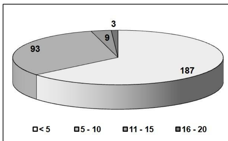
Fig. 9, Frecvența absolută pe clase de valori a duratei intervalelor simultane cu temperaturi tropicale și fără precipitații, din anotimpul de vară (1961-2009), în Câmpia Olteniei.
