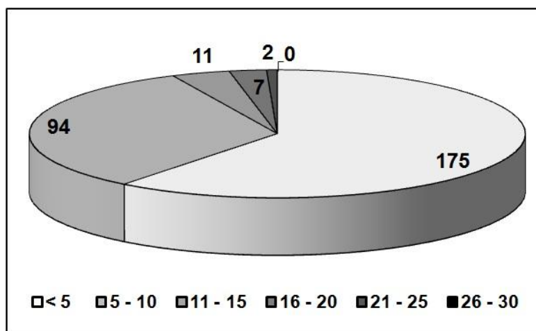
Fig. 6, Frecvența absolută pe clase de valori a duratei intervalelor de zile consecutive cu temperaturi tropicale din lunile de vară, în Câmpia Olteniei (1961-2009).
