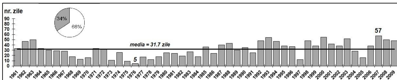
Fig. 5, Variația numărului de zile cu temperaturi tropicale în anotimpul de vară și proporția acestora din totalul zilelor calendaristice (1961-2009), în Câmpia Olteniei.
