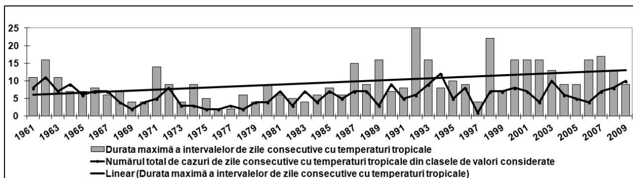
Fig. 7, Variația intervalelor de zile consecutive cu temperaturi tropicale din anotimpul de vară (1961-2009).
