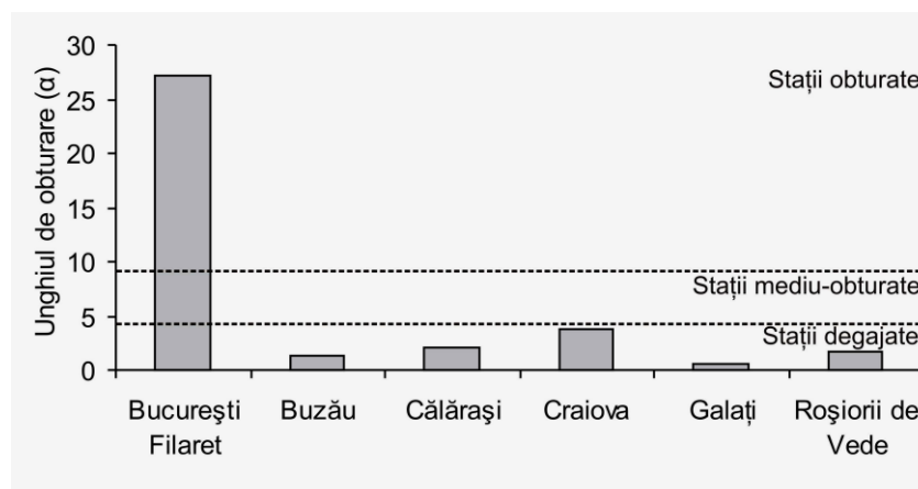
Fig. 1. Unghiul de obturare ( \alpha ) pentru platformele stațiilor meteorologice din Câmpia Română.
