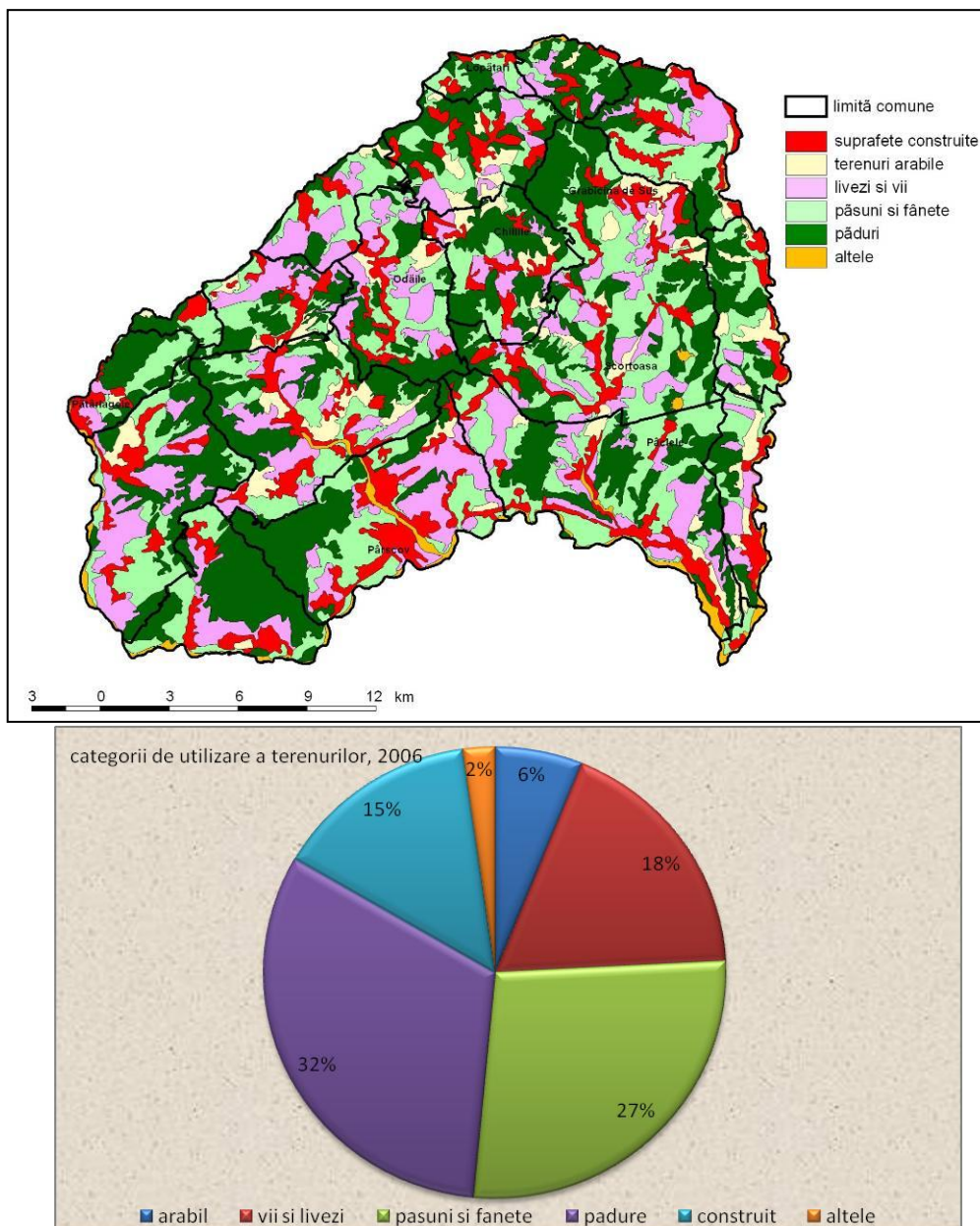
Fig.1. Utilizarea terenurilor în sectorul subcarpatic dintre Buzău și Slănicul Buzăului, 2006 și Ponderea principalelor categorii de utilizare a terenurilor, 2006
