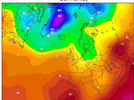
Fig. 2c, Temperatura (°C) la 850 hPa (8500 m), 13.10.1998, ora 00 GMT (din arhiva Centrului Meteorologic Karlsruhe, Germania)
