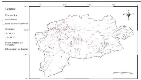
Figure 4. Carte de fracturation et de sismicité de la W. de Guelma.
