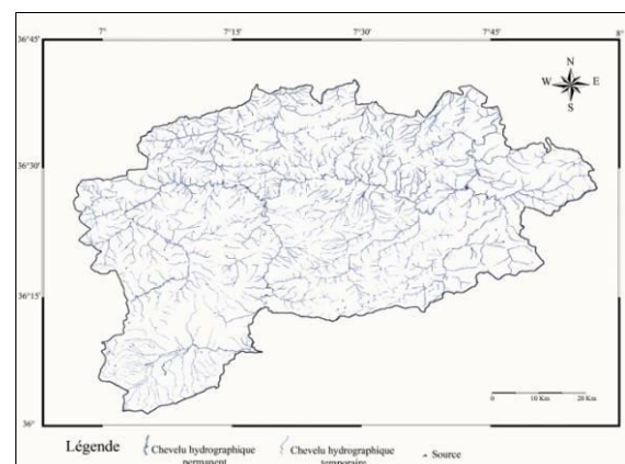
Figure 2. Carte hydrographique de la Wilaya de Guelma
