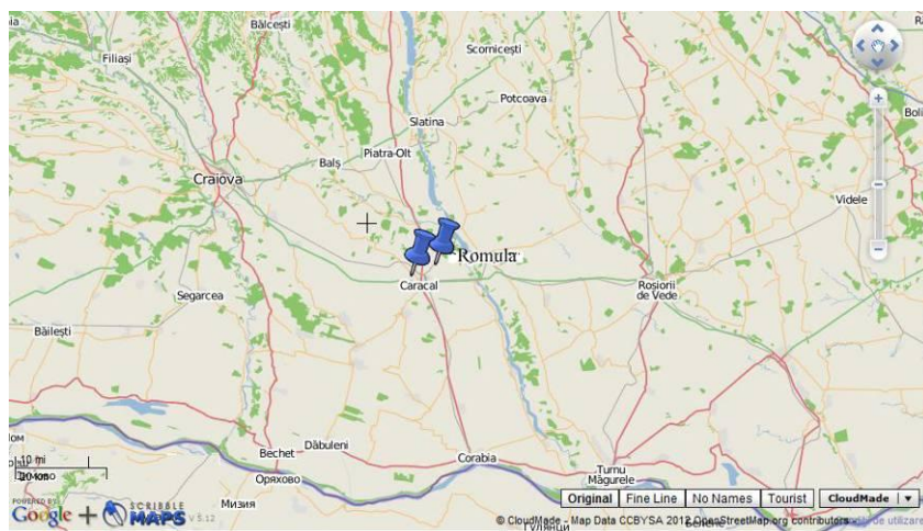
Fig. 1. Amplasarea pe hartă a Romulei
