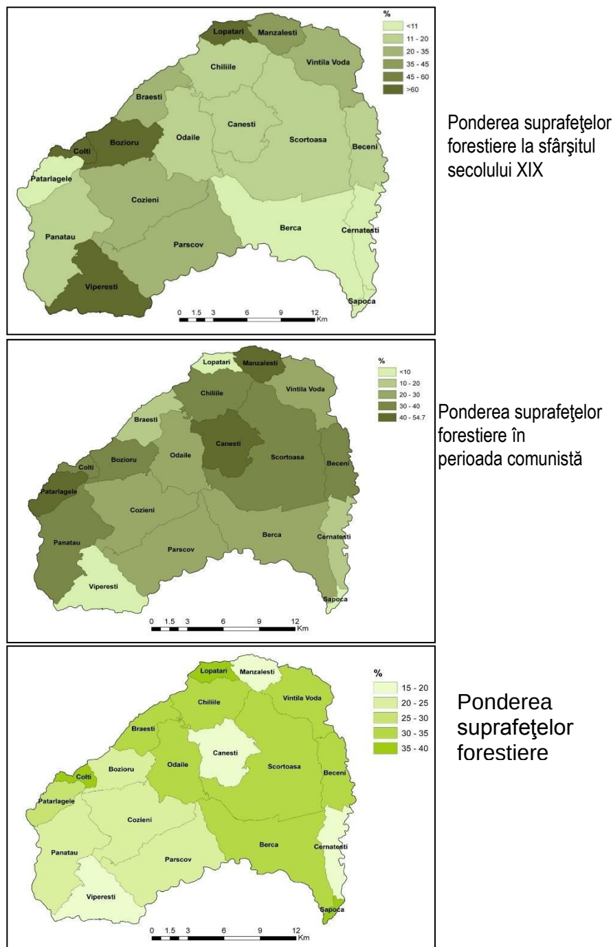
Fig. 2. Pondere suprafețelor forestiere în diferite perioade analizate
