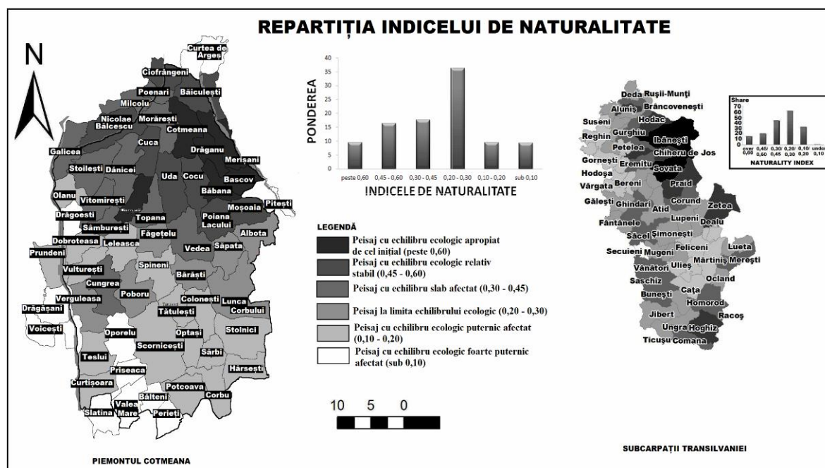
Fig. 5 - Repartiția indicelui de naturalitate în Subcarpații Transilvaniei și în Piemontul Cotmeana – 2011
