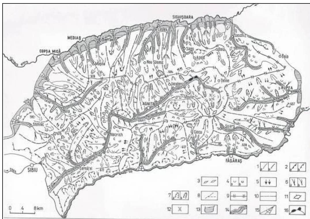
Fig. 2. Podișul Hârtibaciului – Harta proceselor geomorfologice actuale: 1, abrupturi până la 10 m (a, active; b, fixate); 2, abrupturi între 10 și 25 m (a, active; b, fixate); 3, monticuli (glimee); 4, alunecări profunde (2-5 m grosimea materialului deplasat); 5, eroziune în suprafață; 6, ogașe (2-5 m: a, active; b, fixate); 7, ravene (>5 m: a, active; b, fixate); 8, vâlcea, organism torential; 9, culmi cu mameloane și șei; 10, culmi netezite; 11, martor de eroziune; 12, înșeuare; 13, terase; 14, lunci; 15, conuri de dejecție; 16, lacuri artificiale.
