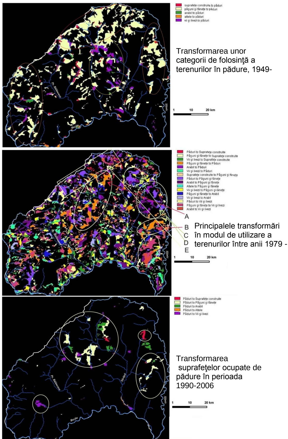
Fig. 3. Principalele transformări în modul de utilizare a terenurilor în trei perioade analizate
