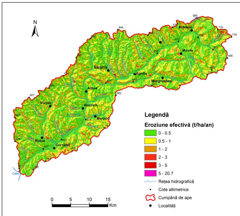
Fig. 3. Harta eroziunii efective.
