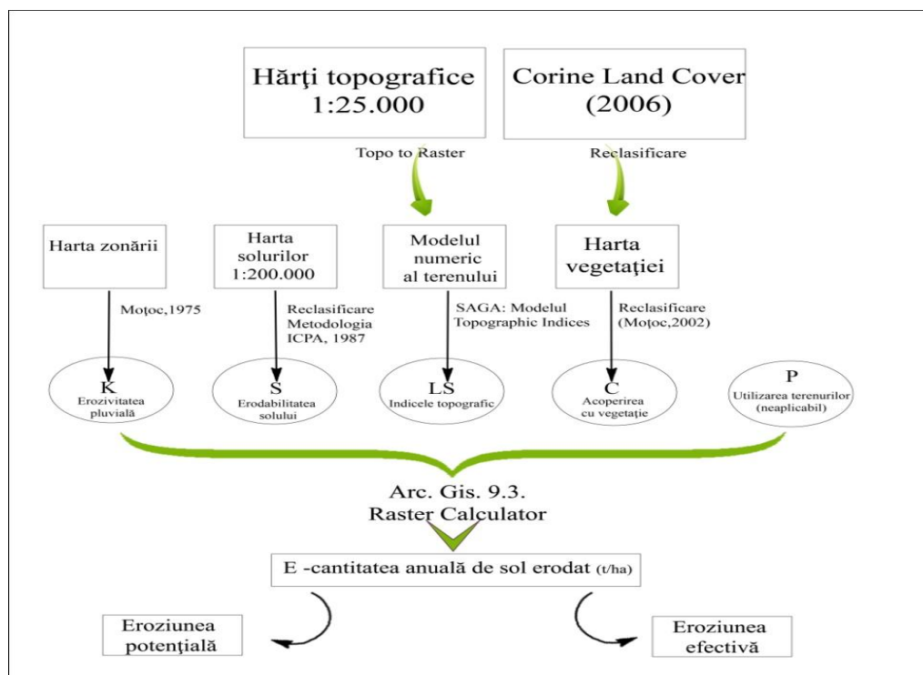
Fig. 2. Metodologia utilizată în elaborarea hărților (după Alexandru și colab., 2012).
