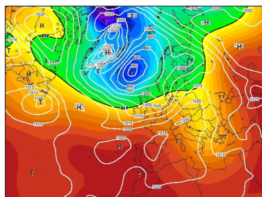
Fig. 2b, Câmpul presiunii atmosferice la sol și câmpul de geopotential la 500 hPa (5500 m), 14.10.1998, ora 00 GMT (din arhiva Centrului Meteorologic Karlsruhe, Germania)
