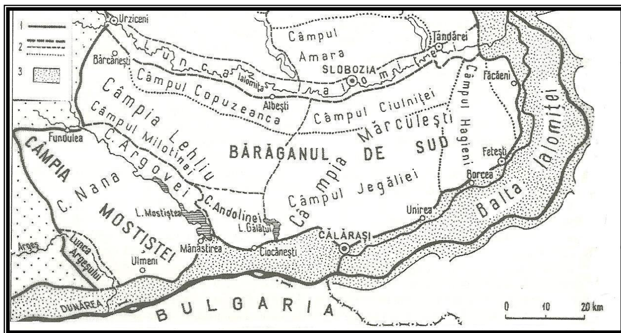
Fig.1 Bărăganul Sudic (După Geografia României, vol. V, 2005 )
