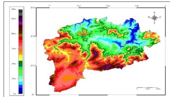
Figure 5. Carte hypsométrique de la W. de Guelma
