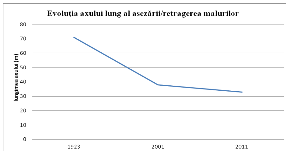
Fig. 3 - Graficul retragerii malurilor lacului între 1923-2011, cu deteriorarea așezării neolitice de la Sultana
