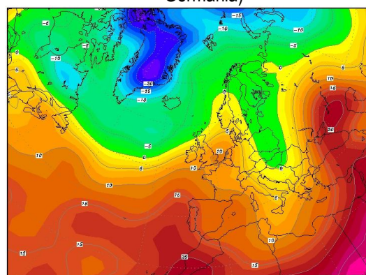
Fig. 2d, Temperatura (°C) la 850 hPa (8500 m), 14.10.1998, ora 00 GMT (din arhiva Centrului Meteorologic Karlsruhe, Germania)
