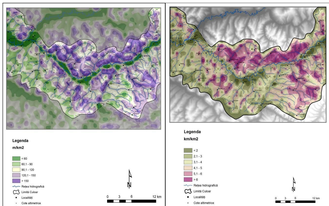
Fig. 2. Harta energiei de relief (stânga) și a fragmentării reliefului (dreapta)
