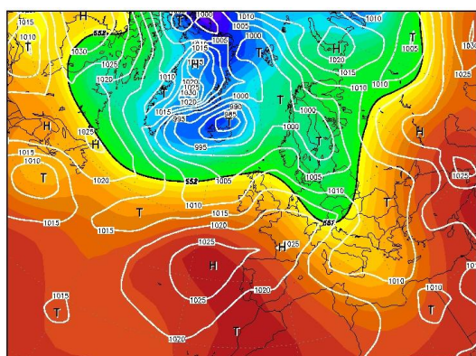
Fig. 2a, Câmpul presiunii atmosferice la sol și câmpul de geopotential la 500 hPa (5500 m), 13.10.1998, ora 00 GMT (din arhiva Centrului Meteorologic Karlsruhe, Germania)
