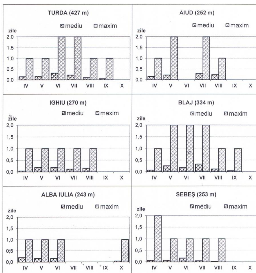
Fig. 1: a, Numărul mediu și maxim anual de zile cu grindină; b, Numărul mediu și maxim lunar de zile cu grindină
