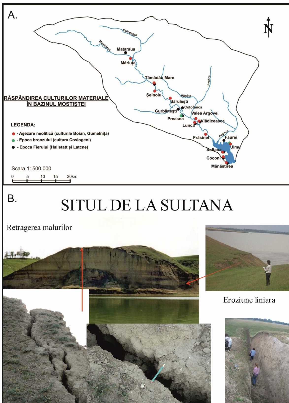
Fig. 1 – Răspândirea culturilor materiale în lungul văii Mostiștea (A) și procese de eroziune a sitului Sultana-Malu Roșu (B)
