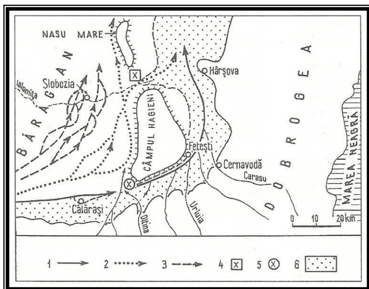
Fig. 3 Captarea Dunării în regiunea Țândărei și Fetești (după Posea Gr. 1984)
